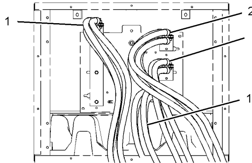
VIEW A-A
